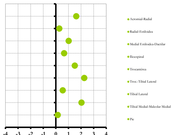
Score-Z Perímetros
