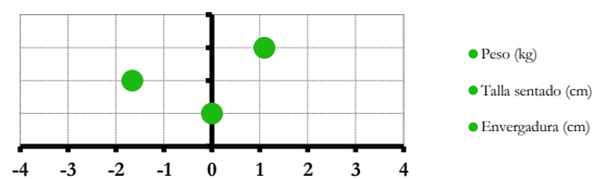
Score-Z Básicos
