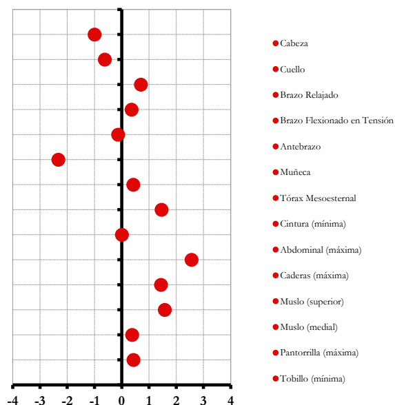
Score-Z Perímetros
